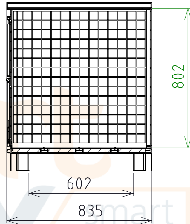
CUT A-A
