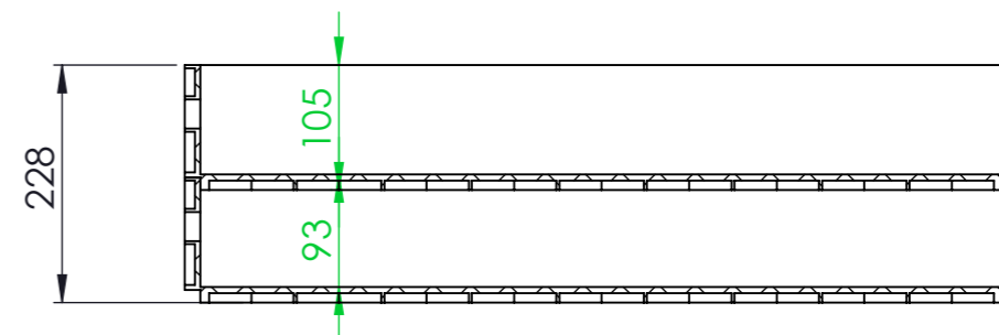
CUT A-A SCALE 1 : 8
