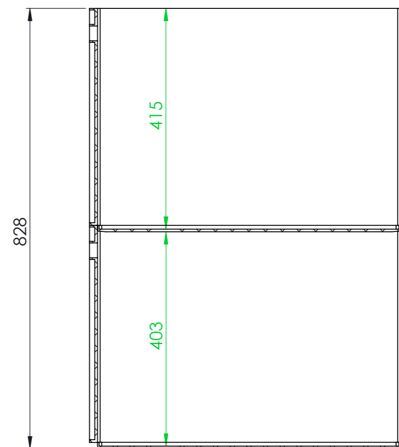
CUT A-A SCALE 1 : 7
