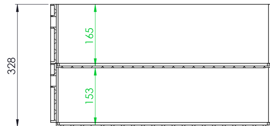
CUT A-A SCALE 1 : 6
