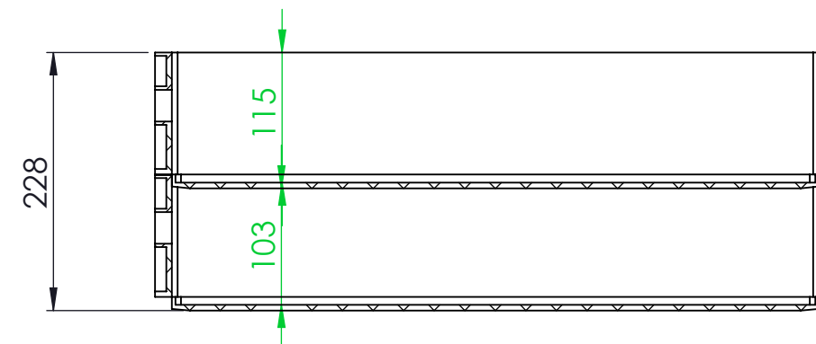
CUT A-A SCALE 1 : 6
