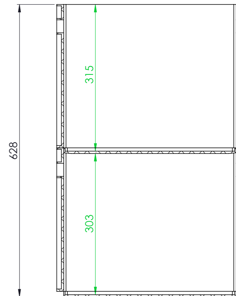
CUT A-A
