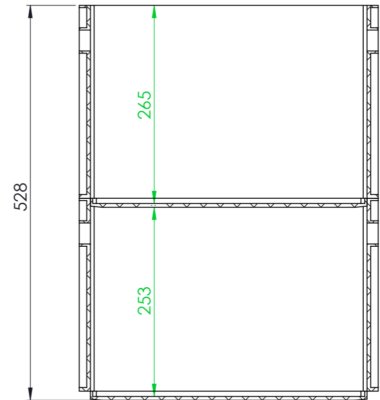
CUT A-A
