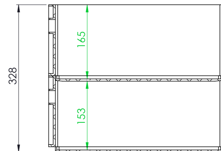
CUT A-A
